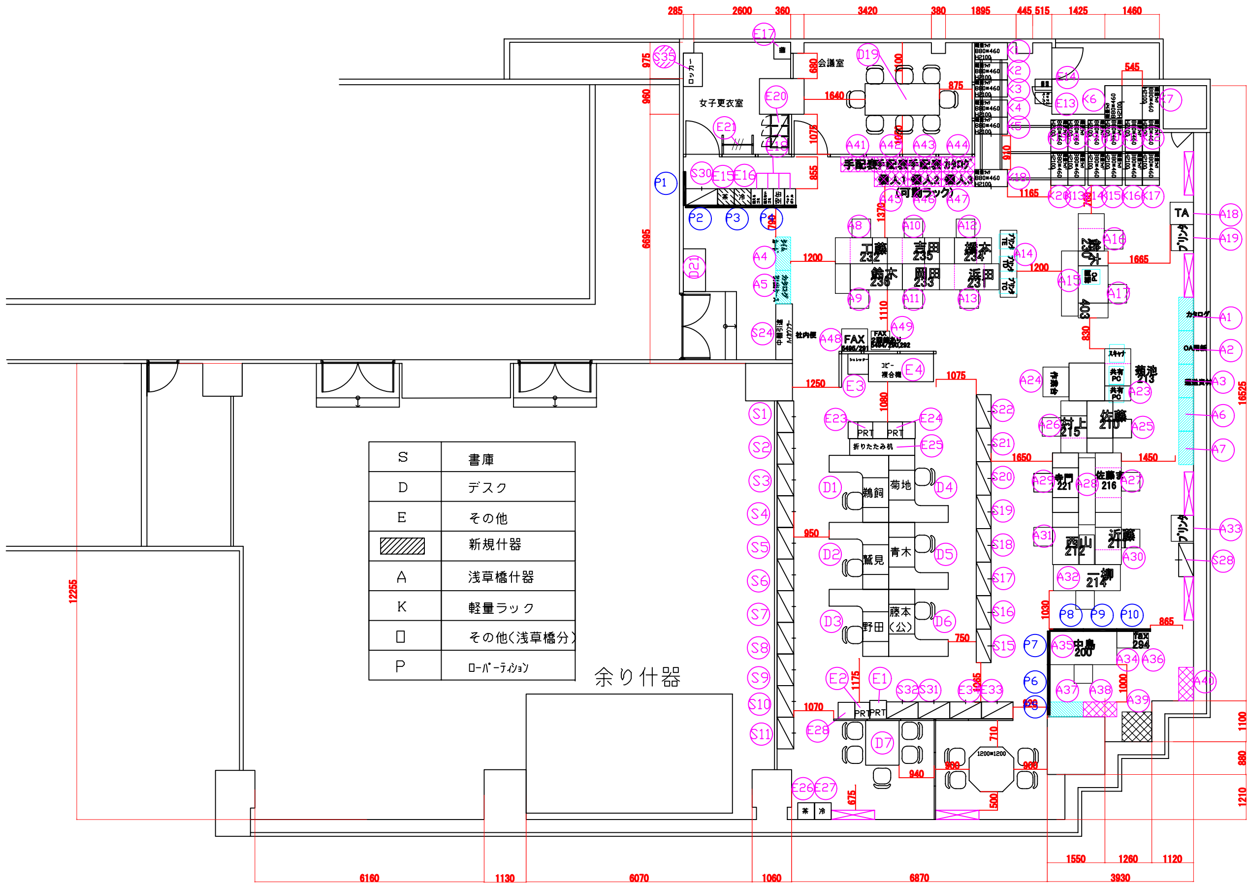
<6F レイアウトプラン>
